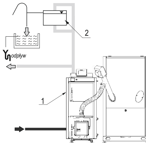
Rysunek 5. Przykładowy schemat zabezpieczeń kotła DELTA EKOPELL: 1-kocioł; 2-otwarte naczynie wzbiornicze.
