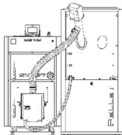
Rysunek 13. Prawidłowe ustawienie zasobnika paliwa względem kotła.
