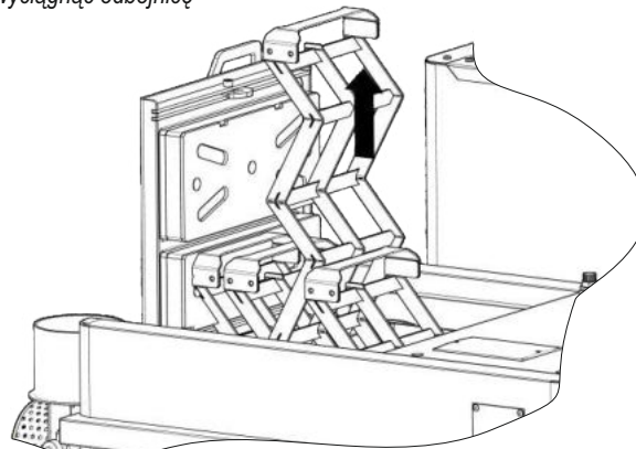
d) wyjąć i oczyścić ekonomizery; ponowny montaż wykonać w odwrotnej kolejności; sprawdzić poprawność montażu Rysunek 16. Sposób czyszczenia zawirowywaczy.
