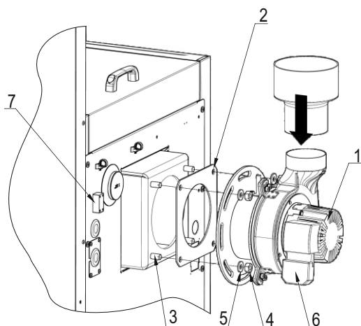
Rysunek 18. Instrukcja montażu wentylatora wyciągowego.
