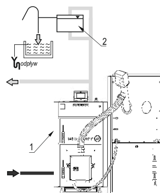
Rysunek 6. Przykładowy schemat zabezpieczeń kotła w układzie otwartym: 1-kocioł, 2-otwarte naczynie wzbiornicze.
