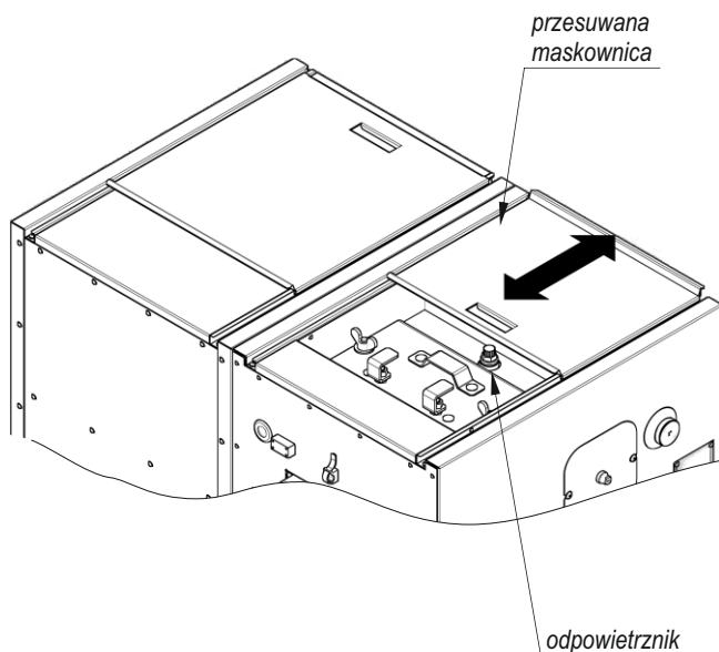
Rysunek 11. Odpowietrznik kotła.
