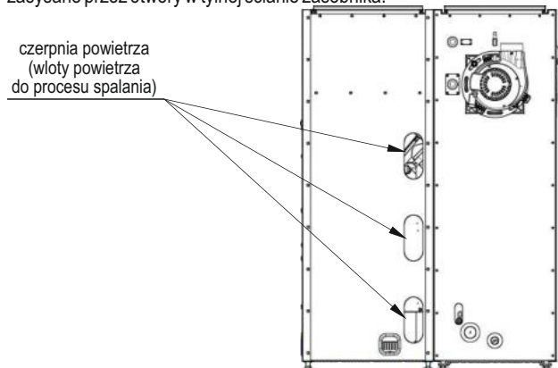
Rysunek 12. Czepnia powietrza - otwory dolotowe powietrza
