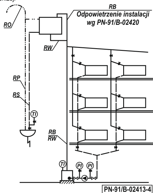
Rysunek 4. Schemat zabezpieczenia instalacji ogrzewania wodnego, wyposażonej w jeden kocioł lub wymiennik ciepła, rozdział górny, pompa zamontowana na powrocie. Schemat zabezpieczenia ma również zastosowanie do następujących instalacji ogrzewania wodnego:
