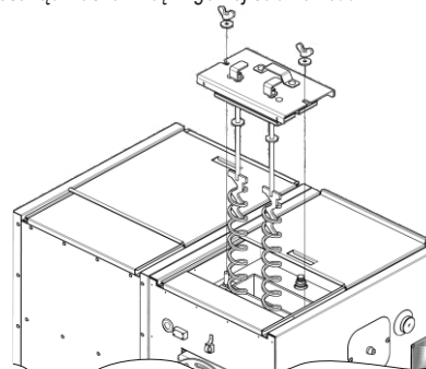
KROK 2. Odkręcić śruby mocujące poręcz wyczystki. Podnieść pokrywę wraz z zawirowywaczami. Oczyszczyć I i II ciąg spalinowy. Zmontować w odwrótej kolejności.
