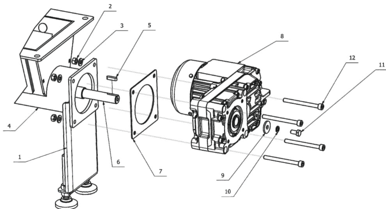
1. Odkręcić śruby M8x90 /poz. 12./ mocujące stopkę regulacyjną rury podajnika /poz. 1./. 2. Wsunąć ślimak /poz. 6./ w rurę podajnika /poz. 4./. 4. Założyć uszczelkę /poz. 7/, nasunąć motoreduktor /poz. 8./ na wałek ślimaka, połączyć za pomocą wpustu /poz. 5./ i przykręcić, motoreduktor razem ze stopką regulacyjną /poz. 1./ do rury podajnika za pomocą dostarczonego śrubunku. 5. Zabezpieczyć /poz. 9.-11./
