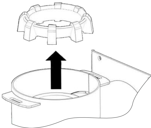
KROK 3. Zdjąć koronę palnika retortowego.
