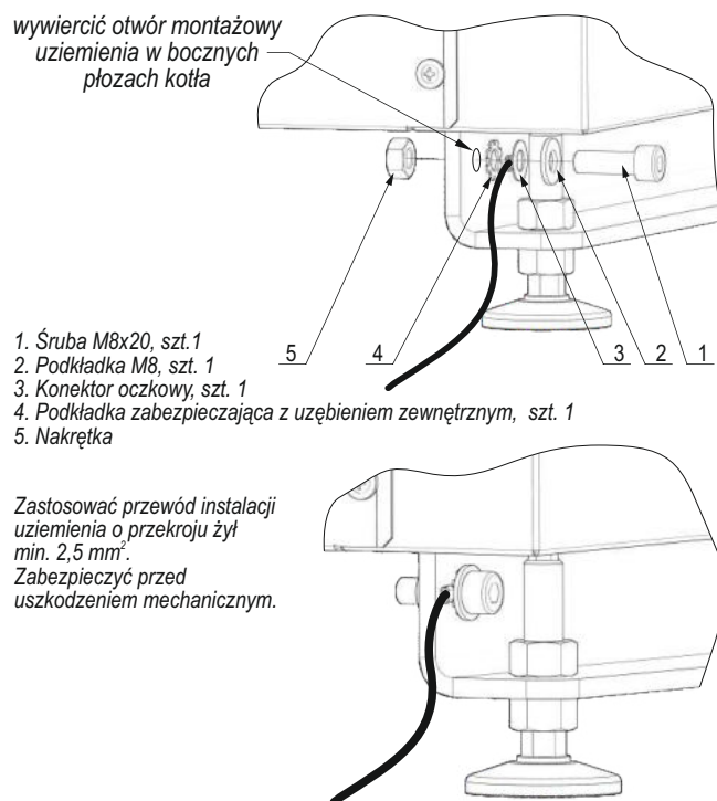
Rysunek 18. Schemat instalacji uziemienia korpusu kotła.
