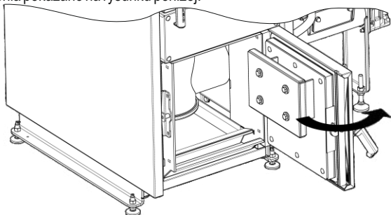
KROK 1. Otworzyć drzwi paleniskowo-popielnikowe.
