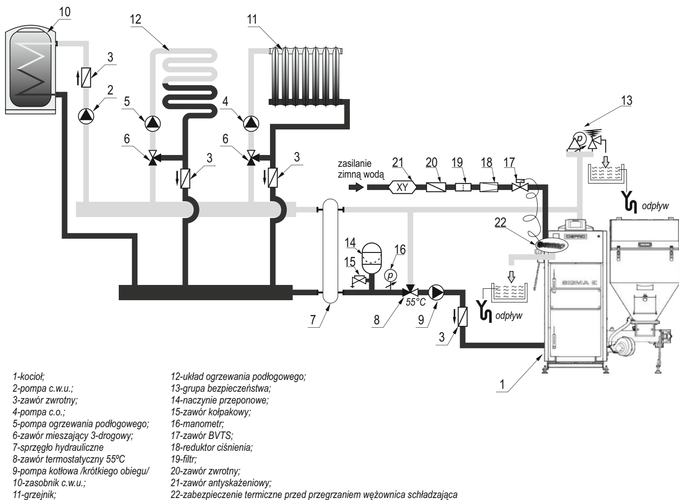
Rysunek 10. Przykładowy schemat instalacji grzewczej systemu zamkniętego.
