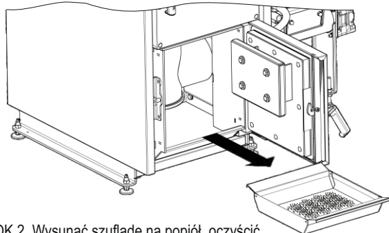
KROK 2. Wysunąć szufladę na popiół, oczyścić.
