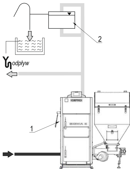
Rysunek 5. Przykładowy schemat zabezpieczeń kotła SIGMA E w układzie otwartym: 1-kocioł; 2-otwarte naczynie wzbiorcze.
