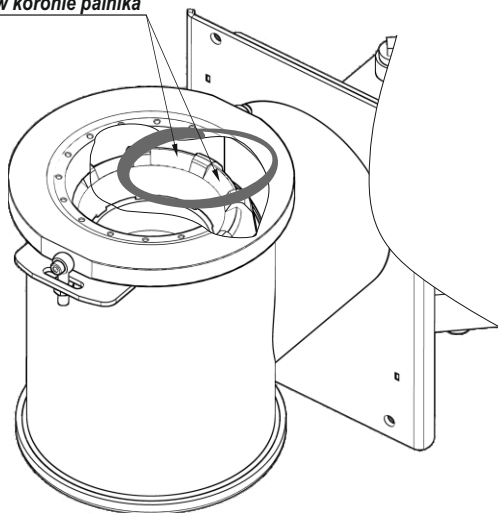
KROK 5. Zmontować palnik retortowy zwracając uwagę, aby przesłona znajdowała się na wprost rury podawczej podajnika.
