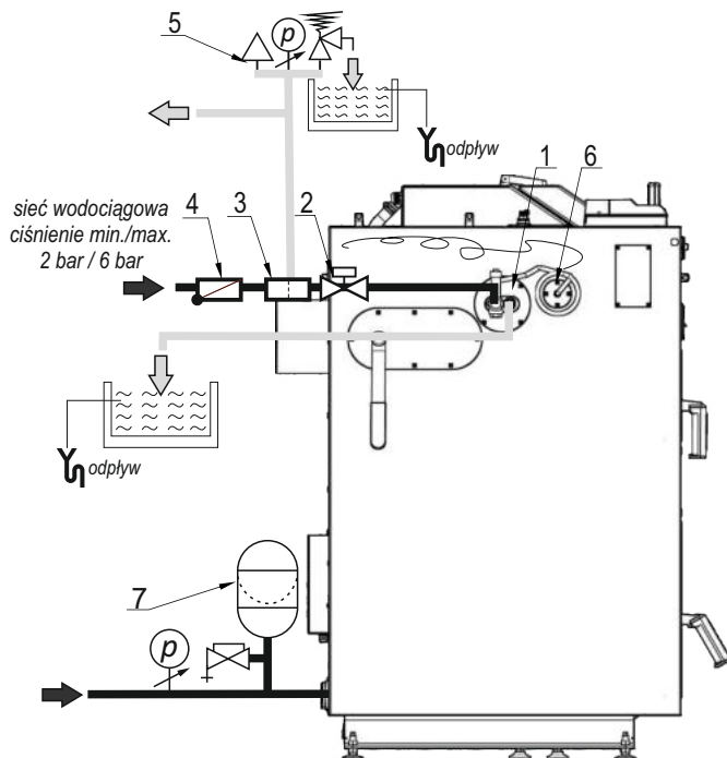
Rysunek 7. Przykładowy schemat zabezpieczeń kotła SIGMA E NZ w układzie zamkniętym: 1-wężownica; 2-zawór BVTs wkręcony w wężownicę; 3-filtr wody użytkowej; 4-zawór zwrotny; 5-armatura bezpieczeństwa; 6-czujnik zaworu BVTs; 7-naczynie wzbiorcze przeponowe.
