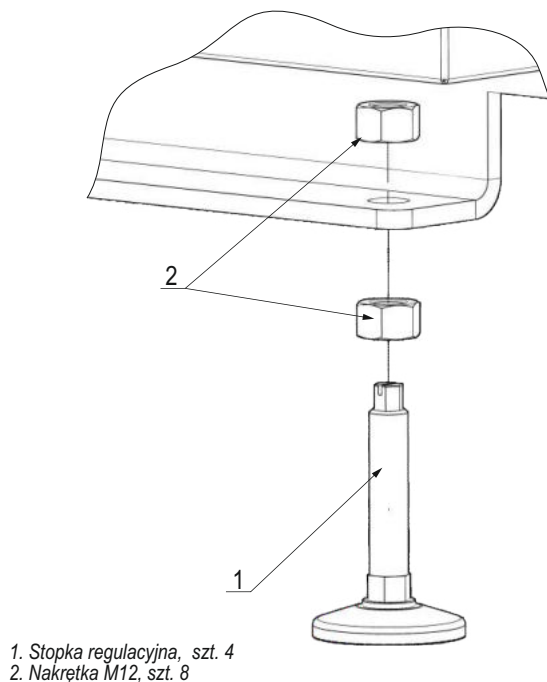
Rysunek 17. Sposób montażu stopek ustalających kocioł.
