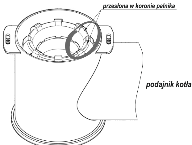
Rysunek 13. Prawidłowe położenie korony palnika retortowego.
