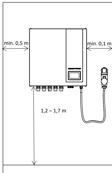
Rys. 3 Montaż hydromodułu.
